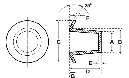
テーパタイプ (SBI1/4, 3/8, 1/2, 3/4のみ)
